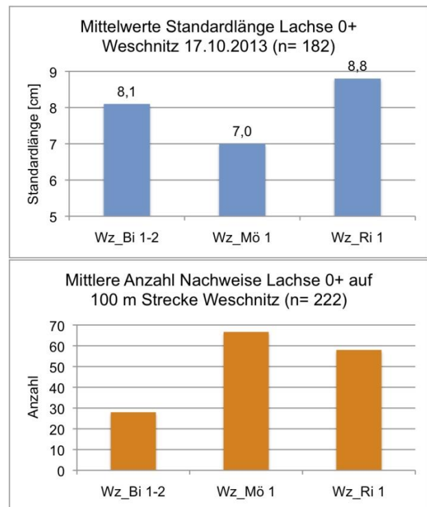
Abb. 15a: Lachse AK 0+ aus drei Probestrecken in der Weschnitz: mittlere Längen (oben) und Nachweise pro 100 m Strecke (unten).
