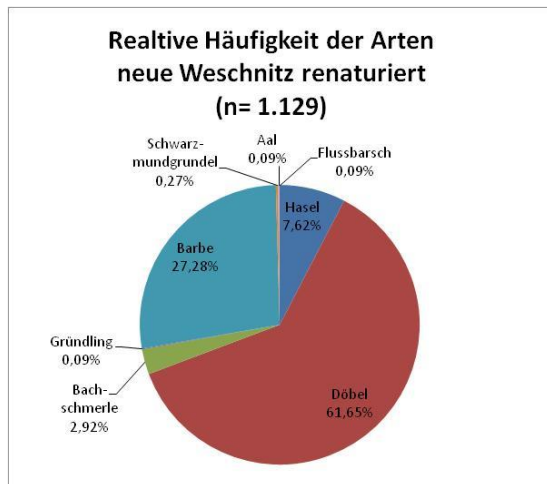
Abb. 19b: Relative Anteile der Fischarten der unteren Weschnitz im Sommer 2020
