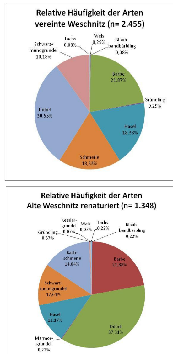
Abb. 19a: Relative Anteile der Fischarten der unteren Weschnitz im Sommer 2020
