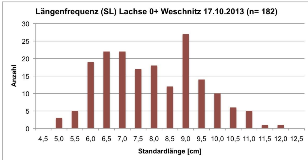
Abb. 15b: Längenfrequenz der Lachse AK 0+ aus drei Probestrecken in der Weschnitz
