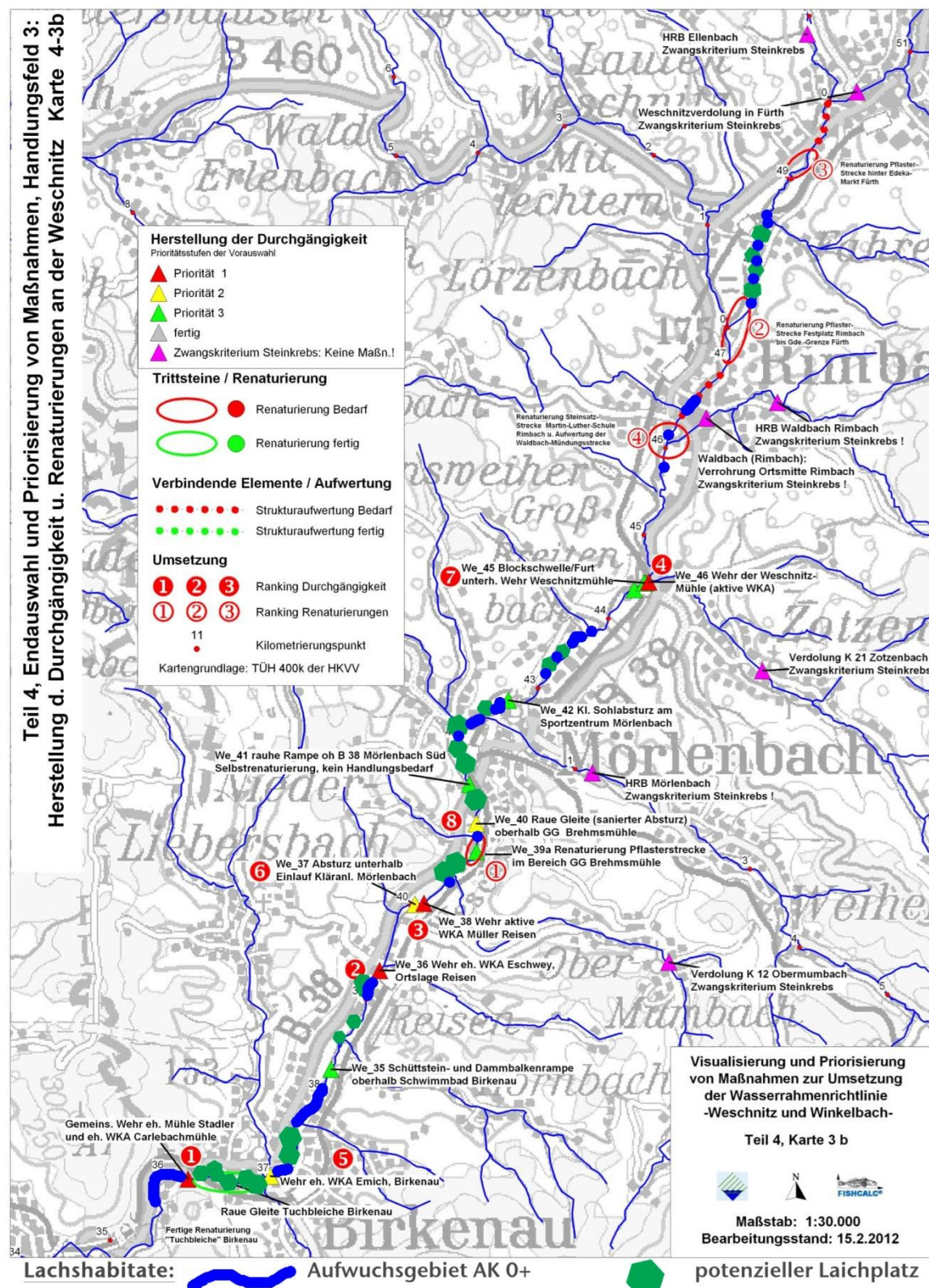
Abb. 2: Laich- und Aufwuchshabitate für den Lachs im Mittellauf der Weschnitz gemäß Begehung/Kartierung 2012 (BFS) (Legende siehe Karte, unten). [Kartengrundlage aus: HENNINGS (2012) „Visualisierung und Priorisierung von Maßnahmen zur Umsetzung der Europäischen Wasserrahmenrichtlinie in den Einzugsgebieten von Weschnitz und Winkelbach - Teil 4: Konkretisierung von Maßnahmen und abschließende Auswahl bzw. Priorisierung “].
