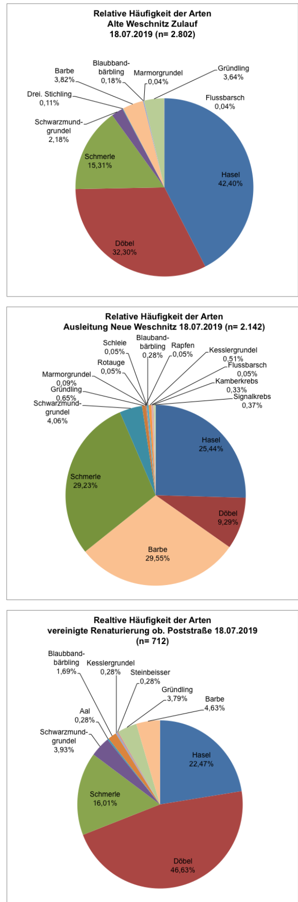
Abb. 17: Relative Anteile der Fischarten der unteren Weschnitz im Sommer 2019
