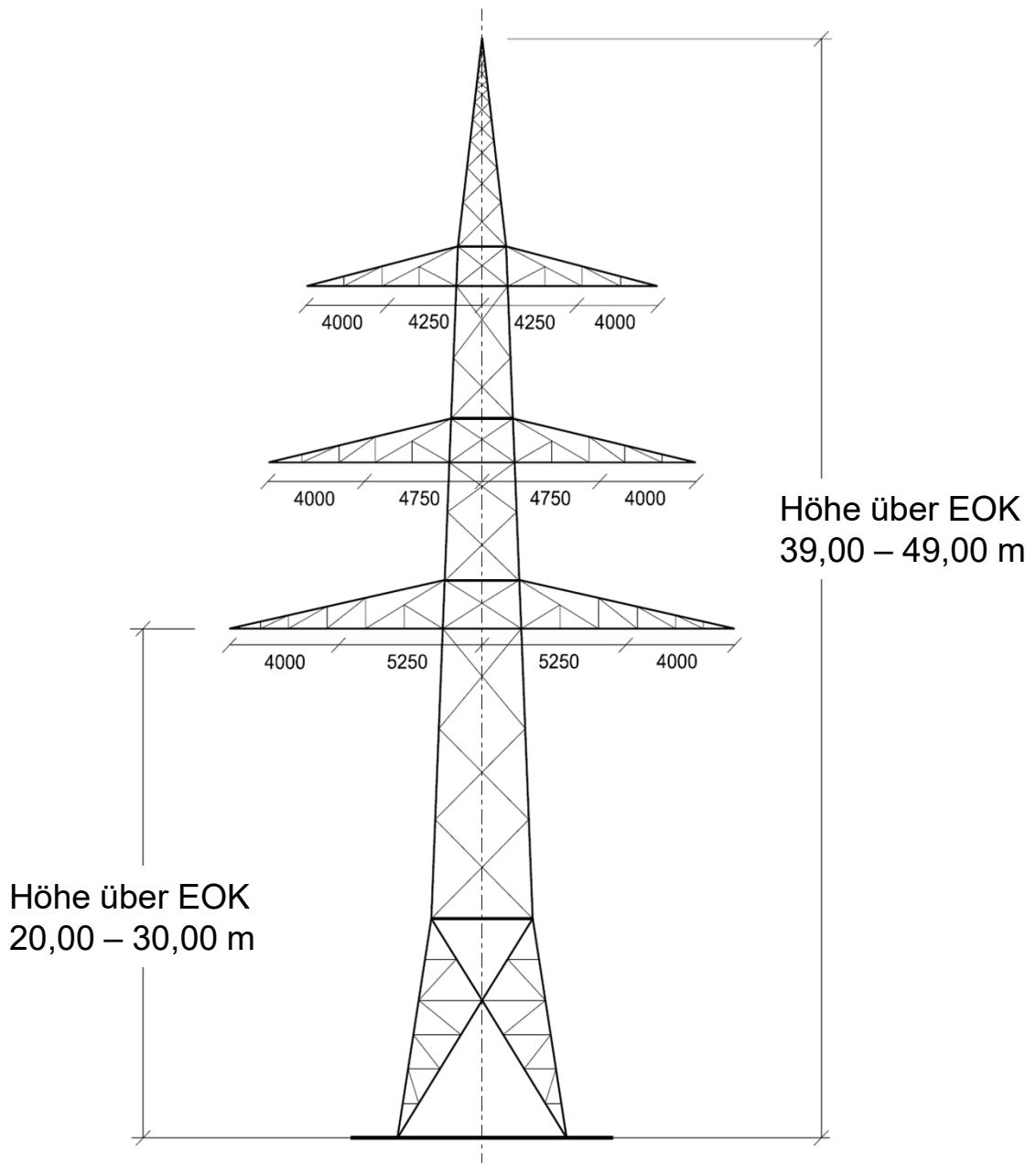
Schemazeichnung (ohne Maßstab) Maßangaben in Millimeter
