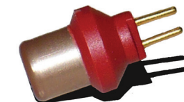
Anzündkerze für Airbag-Gasgenerator
